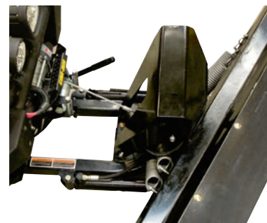
Электрогидравлический блок
