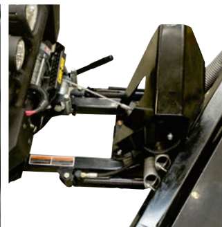
Электрогидравлический блок
